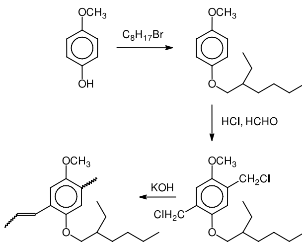
الشكل (9-3): اصطناع بوليمير MEH-PPV 19
